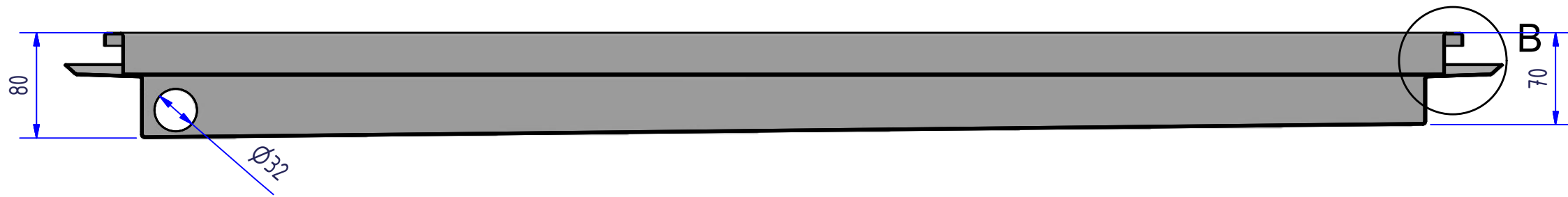
A-A ( 1:4 )
